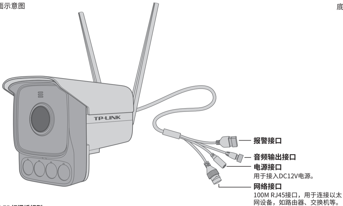
正面示意图
